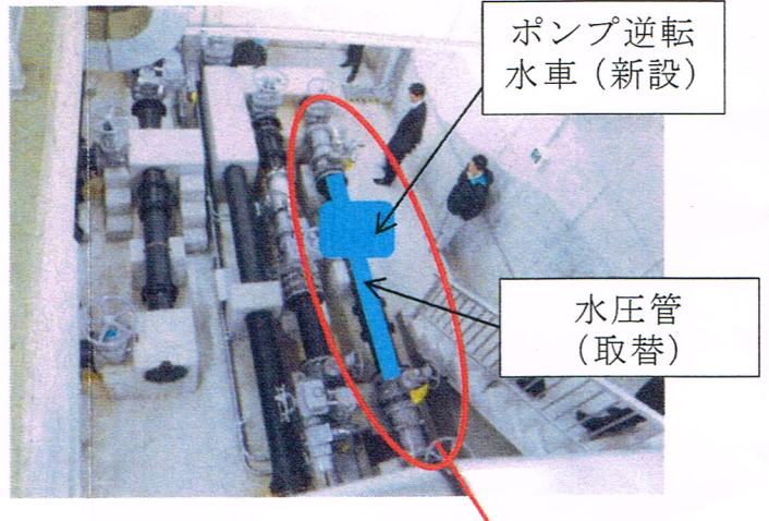
第3減圧槽
